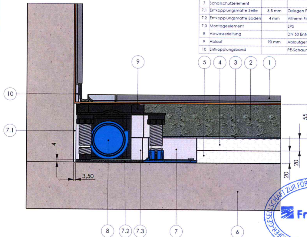
Schnittzeichnung des Prüfaufbaus.
